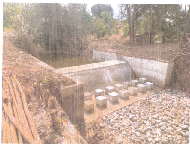
โครงการก่อสร้างพนังป้องกันคอสะพานห้วยสัก บ้านห้วยสัก หมู่ที่ ๙
